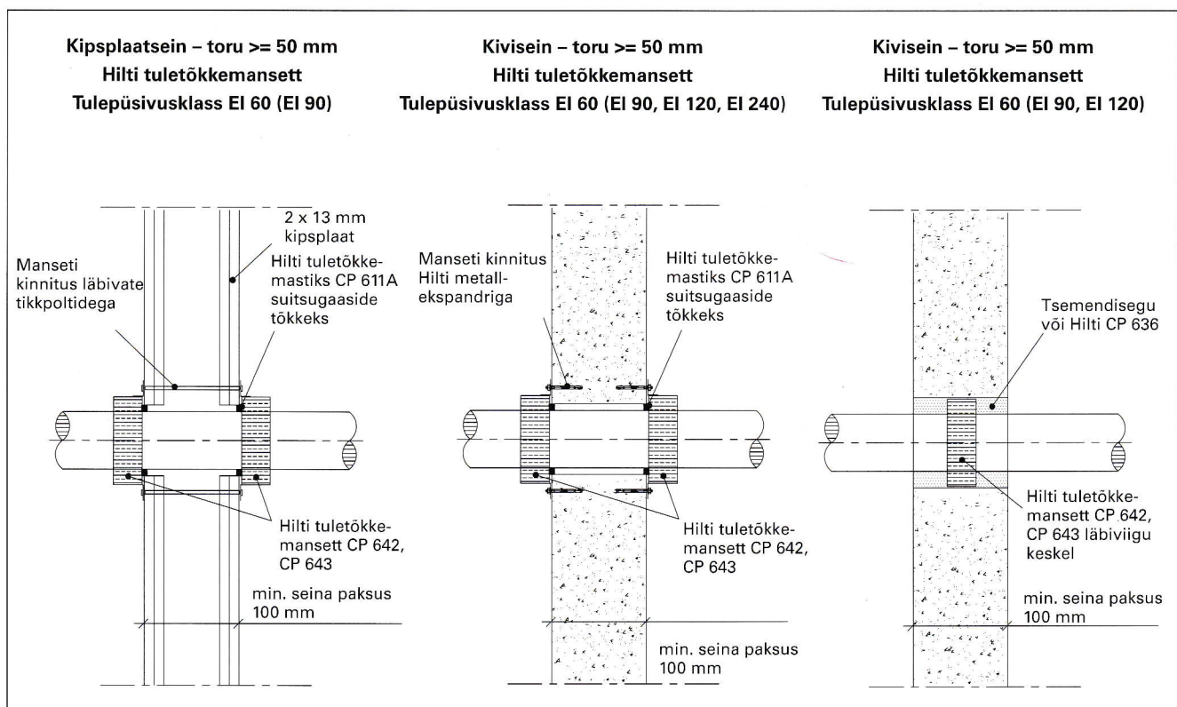
Joonis 6. Seinaläbiviikude näited tuletõkkemansette kasutades.
