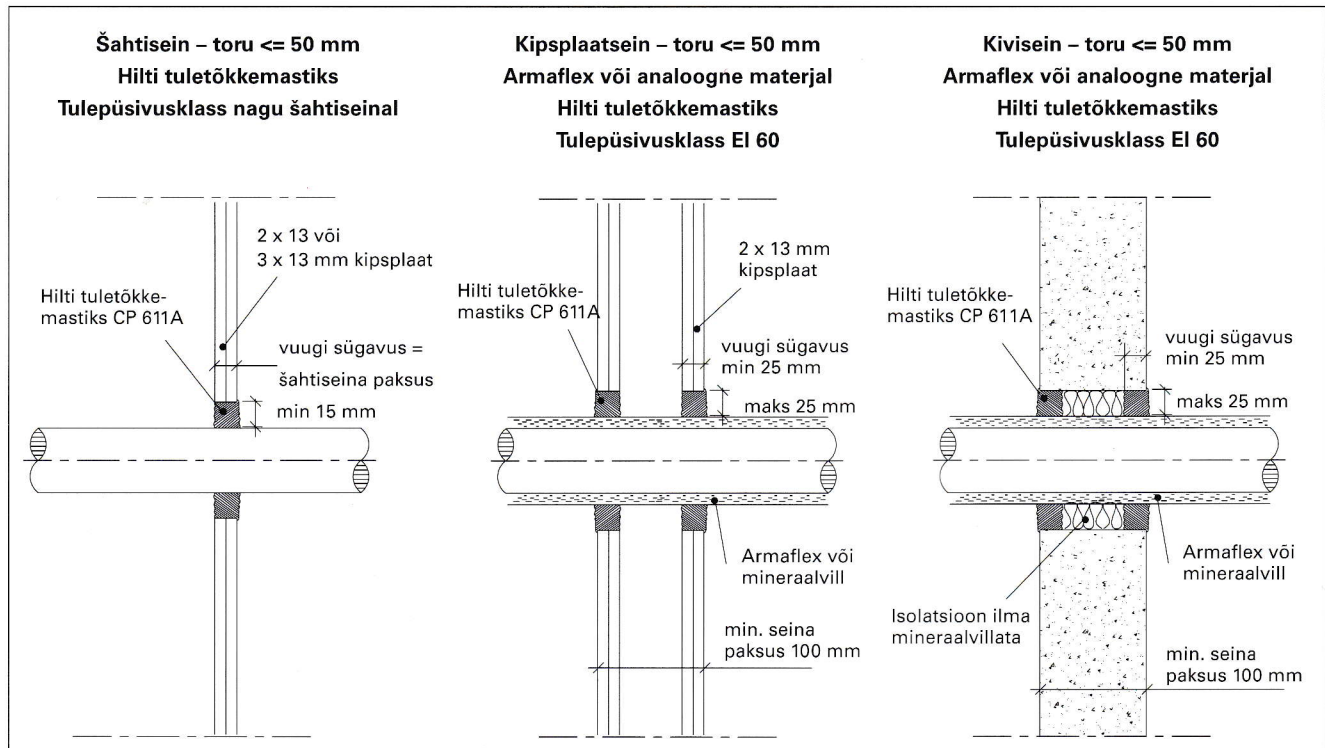
Joonis 5. Seinaläbiviikude näited tuletõkkemastiksit kasutades.
